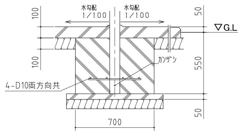
A-A' 断面 1/20
